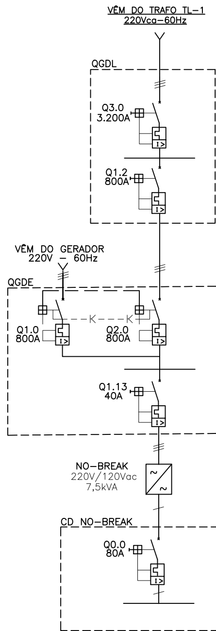
UNIFILAR ALIMENTACAO CD NO-BREAK
